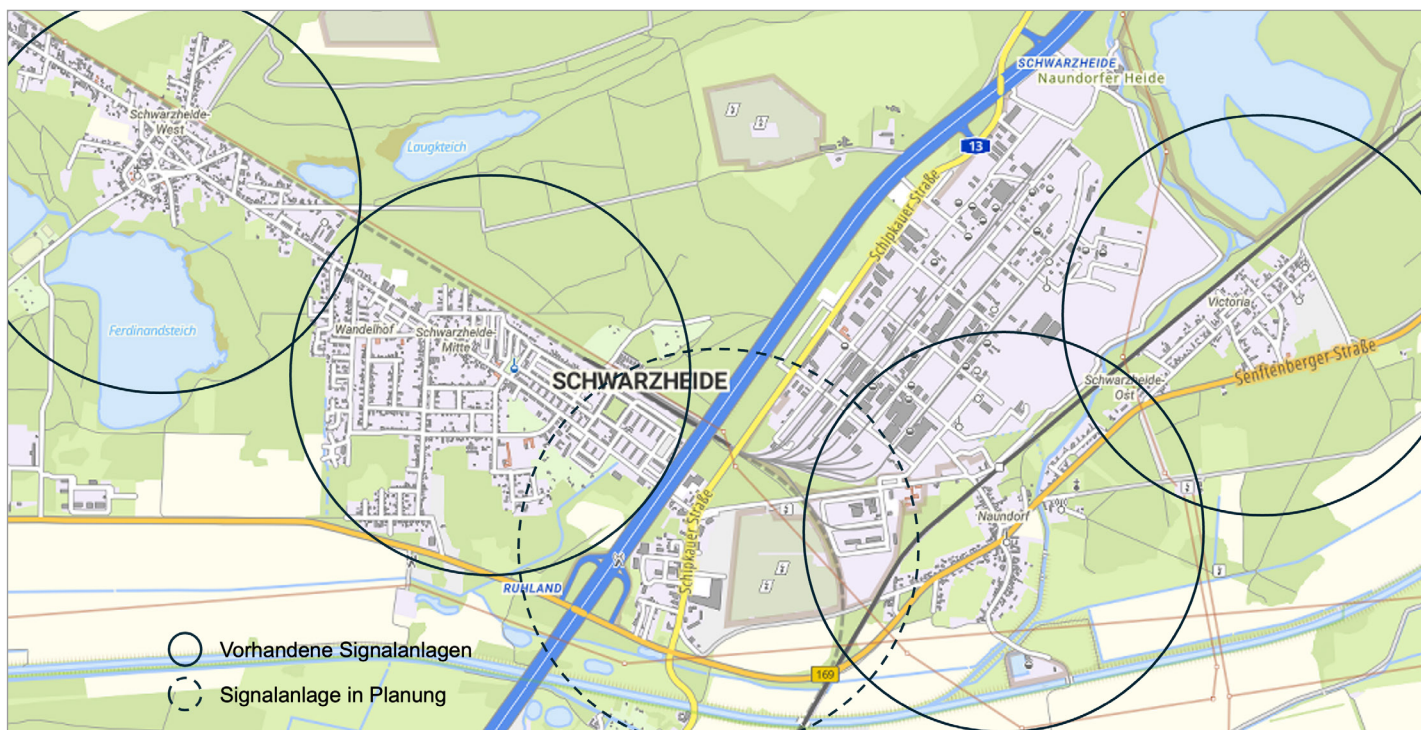
Abbildung: Lautsprecherstandorte und ihre Reichweite
